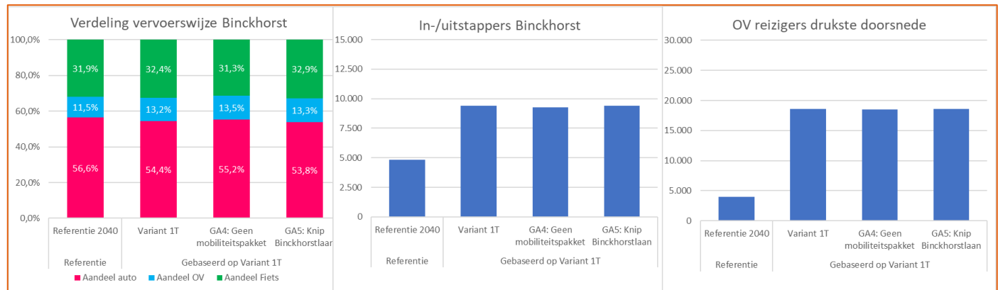
Figuur 6-5 Effecten gevoeligheidsanalyses gericht op lokale maatregelen rond Binckhorst (Brongegevens: Goudappel, 2022)
