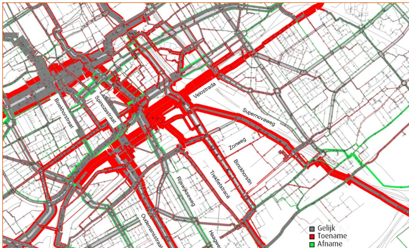
Figuur 3-7 Verschilplot fietsers (etmaal) tussen huidig (2019) en referentie (2040) o.b.v. V-MRDH
