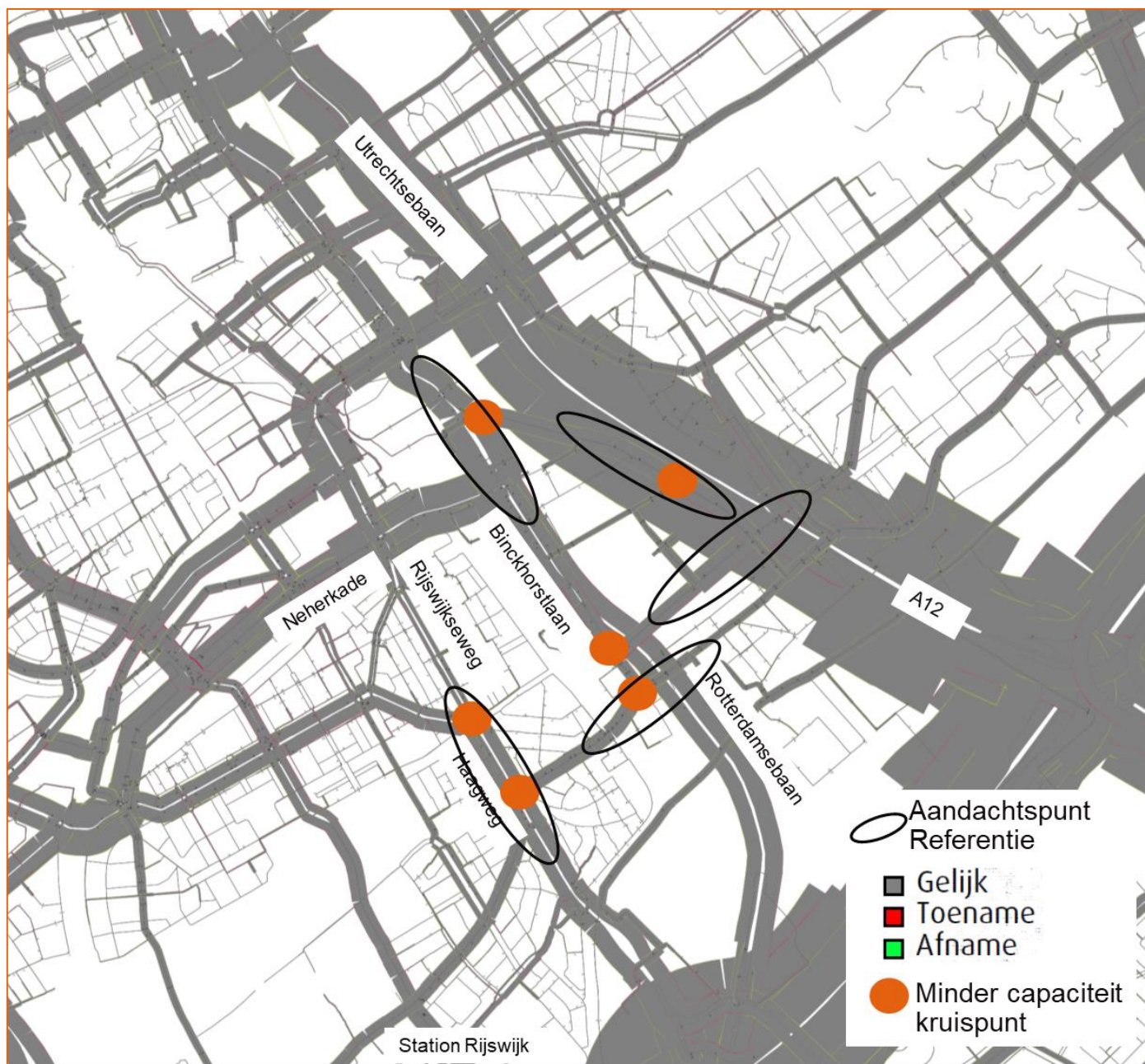
Figuur 4-6 Toe- en afname verkeersintensiteiten tussen Referentie 2040 en alternatieven en aandachtskruispunten
